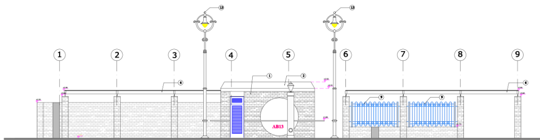
ΔΥΤΙΚΗ ΟΨΗ
