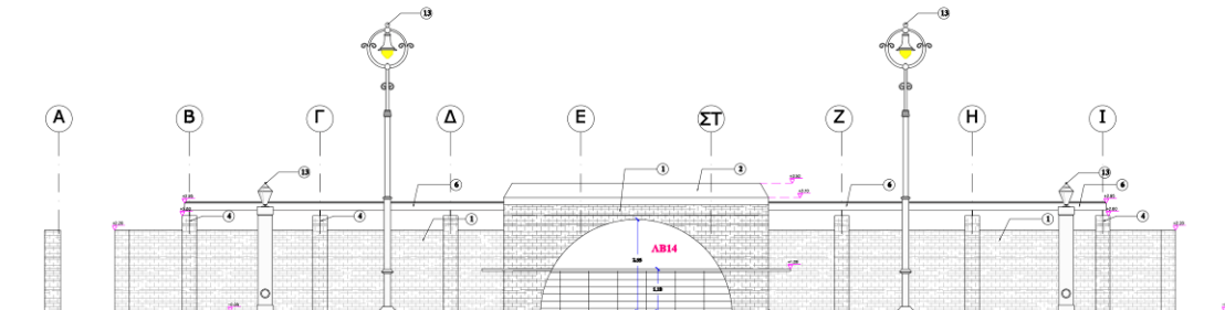
ΝΟΤΙΑ ΟΨΗ
