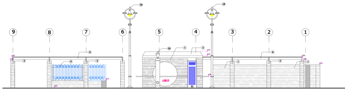
ΑΝΑΤΟΛΙΚΗ ΟΨΗ
