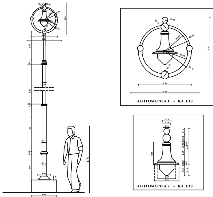
Θ1. ΦΩΤΙΣΤΙΚΟ ΛΙΜΕΝΟΣ ΜΥΚΟΝΟΥ - ΠΑΡΑΔΟΣΙΑΚΟΥ ΤΥΠΟΥ - ΚΛ. 1/20
